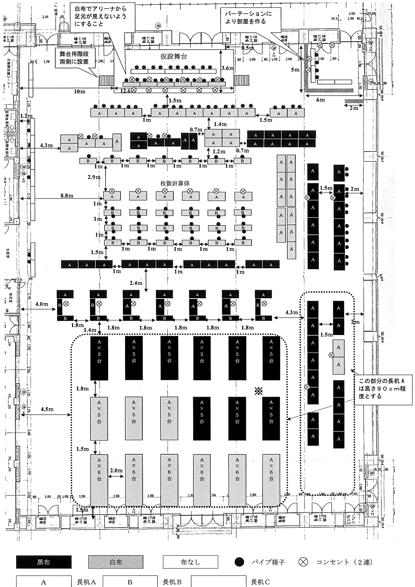
体育館平面図 (49m × 37m)
