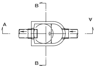
A－A断面図
