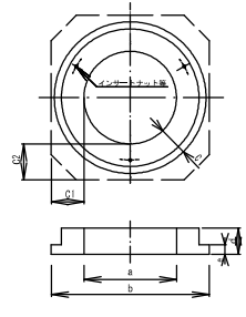
台座 (ふた高さ110mm)
