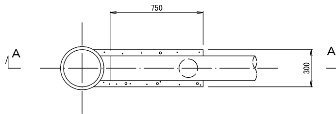
平面图
