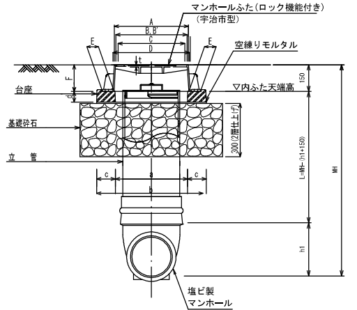
B-B断面図
