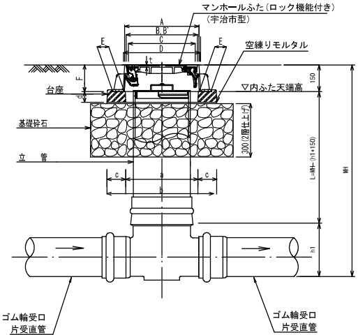
A-A断面図
