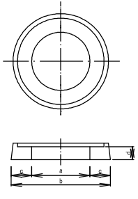
台座 (ふた高さ150mm)
