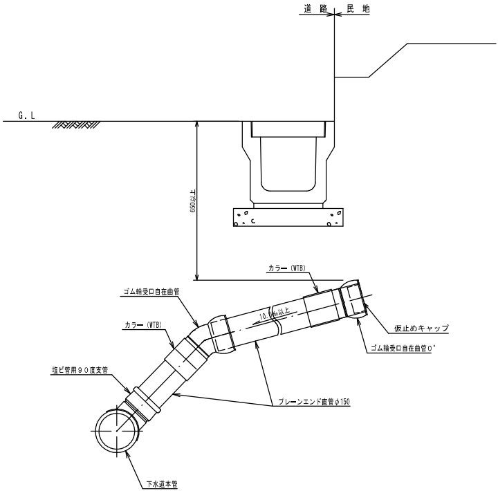
取付管止め標準図
