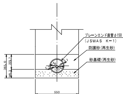
断面図
