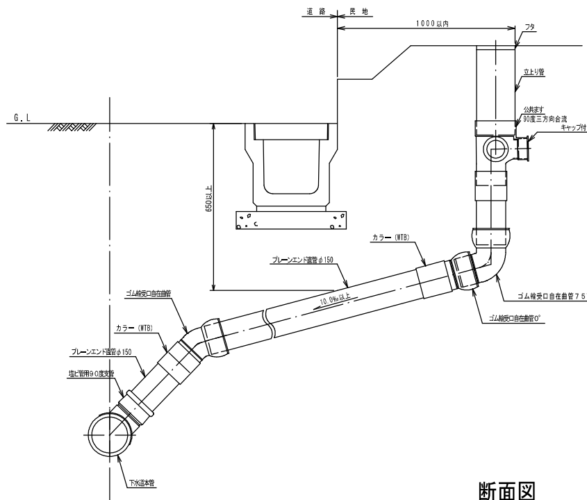
断面図
