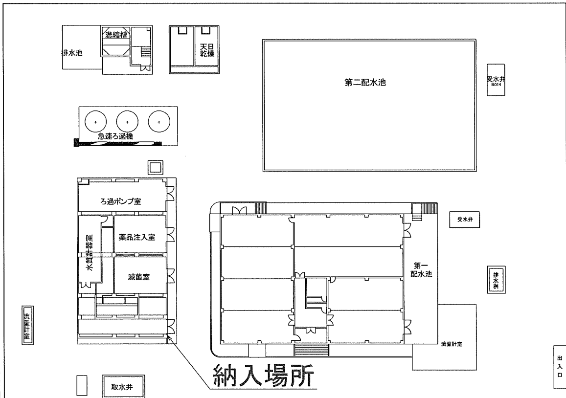
西小倉浄水場全体配置図
