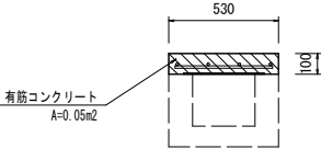
側溝(2) S=1:20
