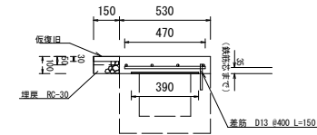
現場打ち床板工300
