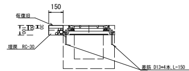
現場打ちグレーチング工30
