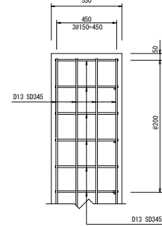
配筋图
