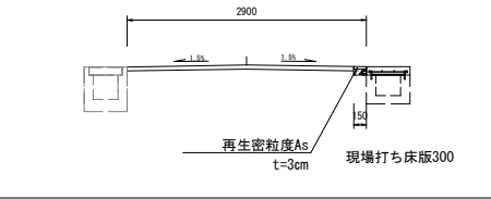
標準横断面図 S=1:50
