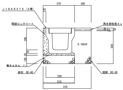
側溝 P U 3 0 0 A
