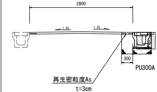
標準横断面図 S=1:50
