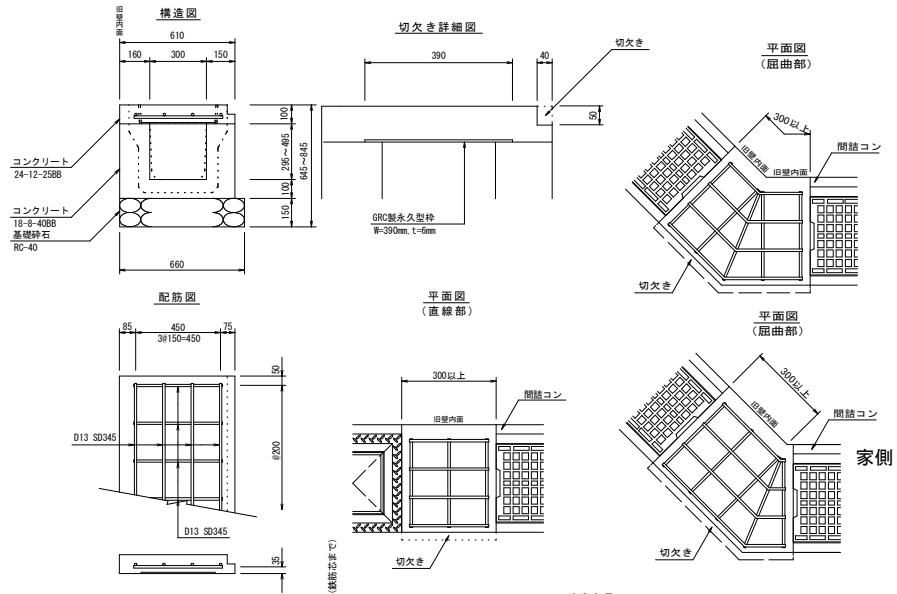
落ちふた式U形側溝3種 取り合い部（間詰コン有）参考図 みぞ幅300の場合
