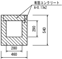
側溝(1) S=1:20
