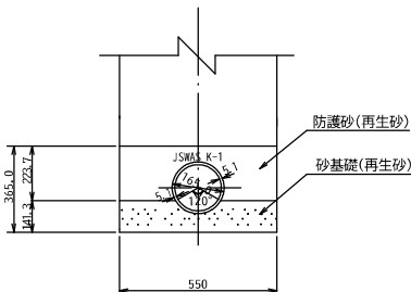
断面図
