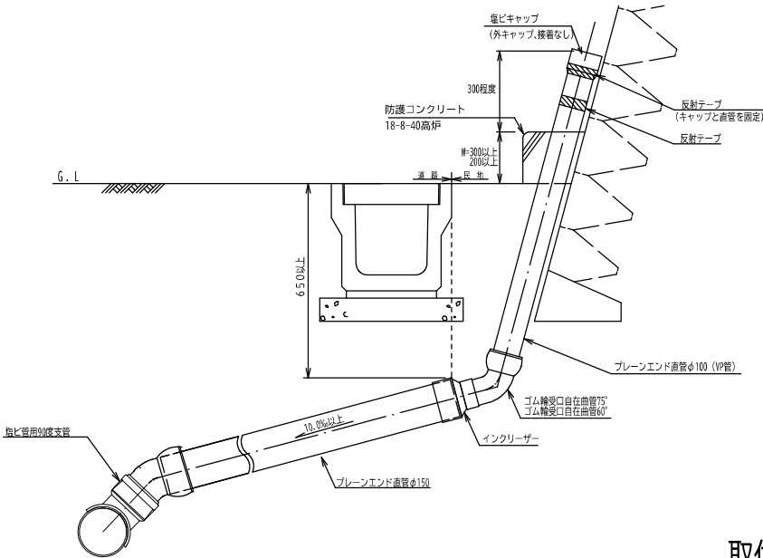
断面図
