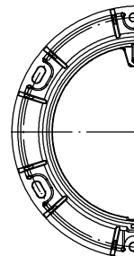
受枠平面図
