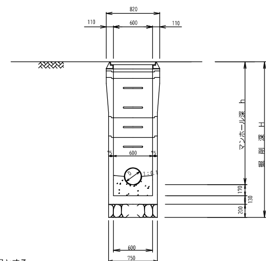
B-B断面図 (方円形・楕円形共通)
