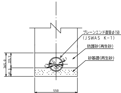
断面図
