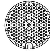
蓋平面図 (スリップ防止型)
