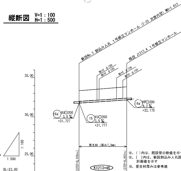
縦断面 V=1:100 H=1:500
