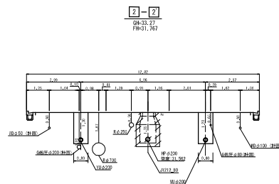
横断面図 S=1:100
