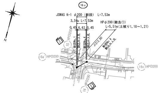
平面図 S=1:500
