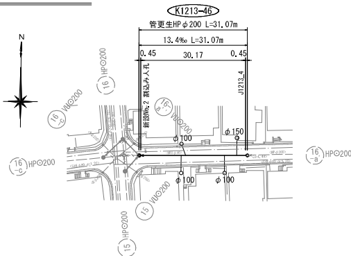
平面図 S=1:500
