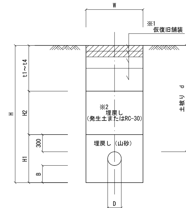
埋戻標準図
