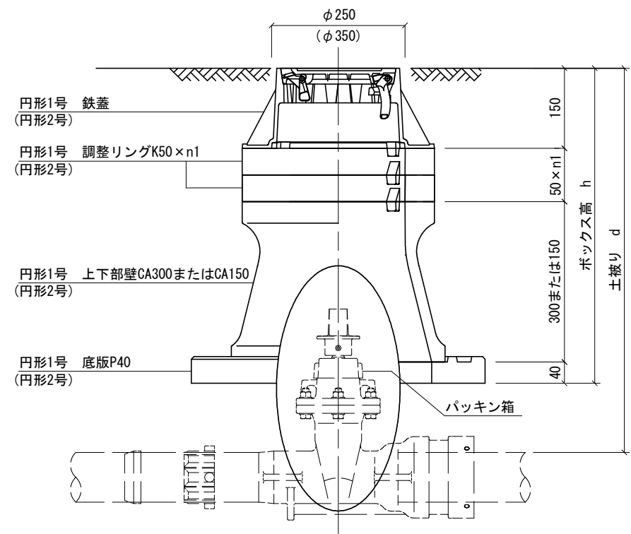
鉄蓋レイアウト例
