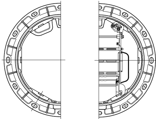
受枠平面図
