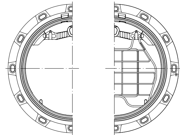
受枠平面図 (次世代型)
