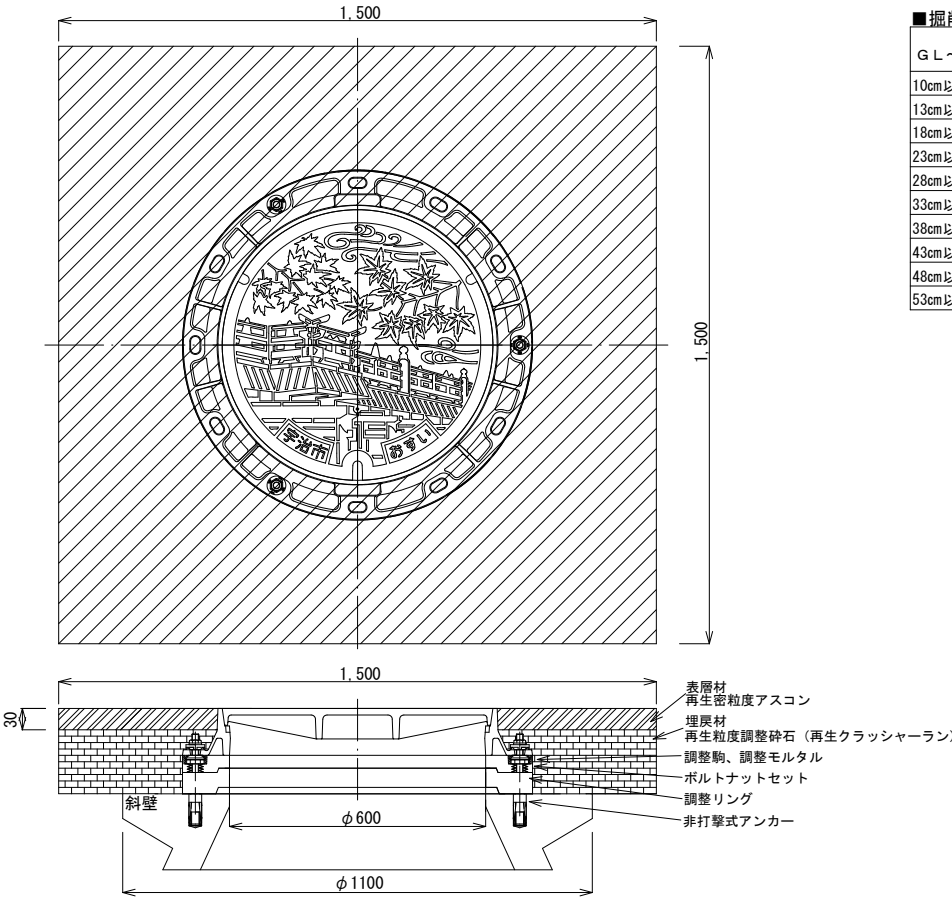
現場打マンホール
