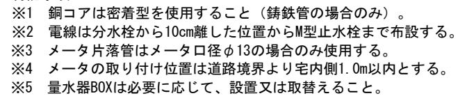
タイプ 1 次 側 2 次 側 サマ付分水栓 (個) 銅77 (個) 伸縮可撓継手 (個) HIP (m) HIL (個) HIS (個) Hユニオン (個) フレキシブル継手2m (個) M型止水栓 (個) メタ片落管 (個) 電線 (m) 表示ビーン (個) 置水器BOX (個) 伸縮継手 (個) HIP (m) HIS (個) φ20 φ25 φ20 φ25 φ20 φ25 φ20 φ25 φ20 φ25 φ20 φ25 φ20 φ25 φ20 φ25 φ20 × φ13 φ13 φ20 φ25 φ13 φ20 φ25 φ13 φ20 φ25 type3-13 1 1 1 L 2 1 1 1 1 1 L+2.0 1 (1) 1 0.3 2 type3-20 1 1 1 L 2 1 1 1 1 L+2.0 1 (1) 1 0.3 2 type3-25 1 1 1 L 2 1 1 1 1 L+2.0 1 (1) 1 0.3 2
