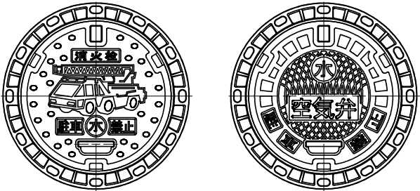
鉄蓋レイアウト例
