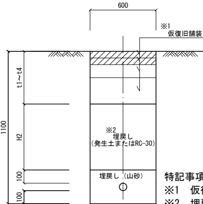
直線部土工断面寸法表
