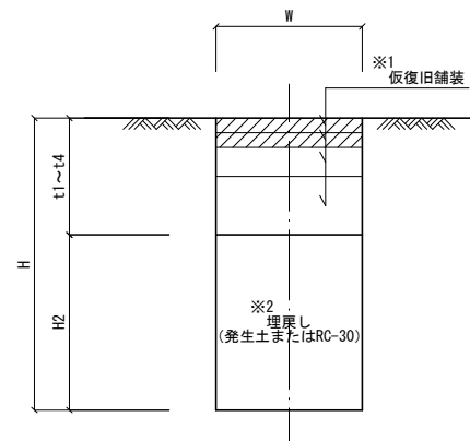
埋戻標準図
