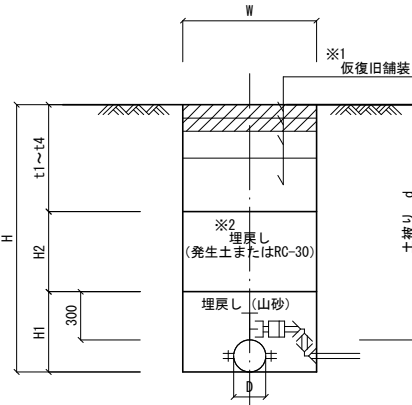
分岐部土工断面寸法表
