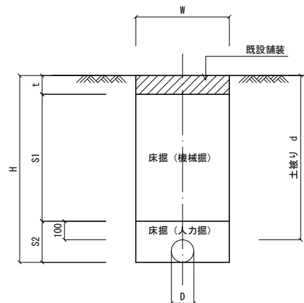
掘削標準図
