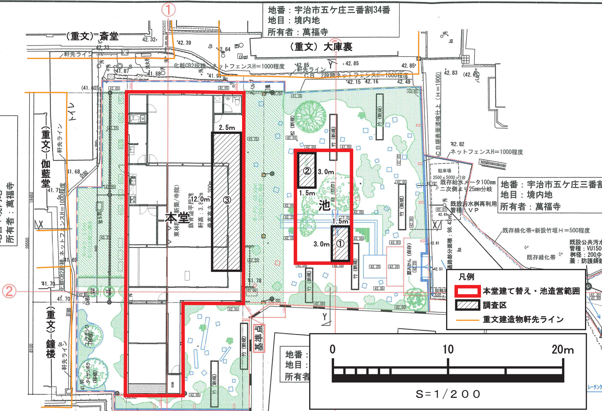
委託内訳 1 (京都府指定史跡萬福寺境内) 調査トレンチ配置図
