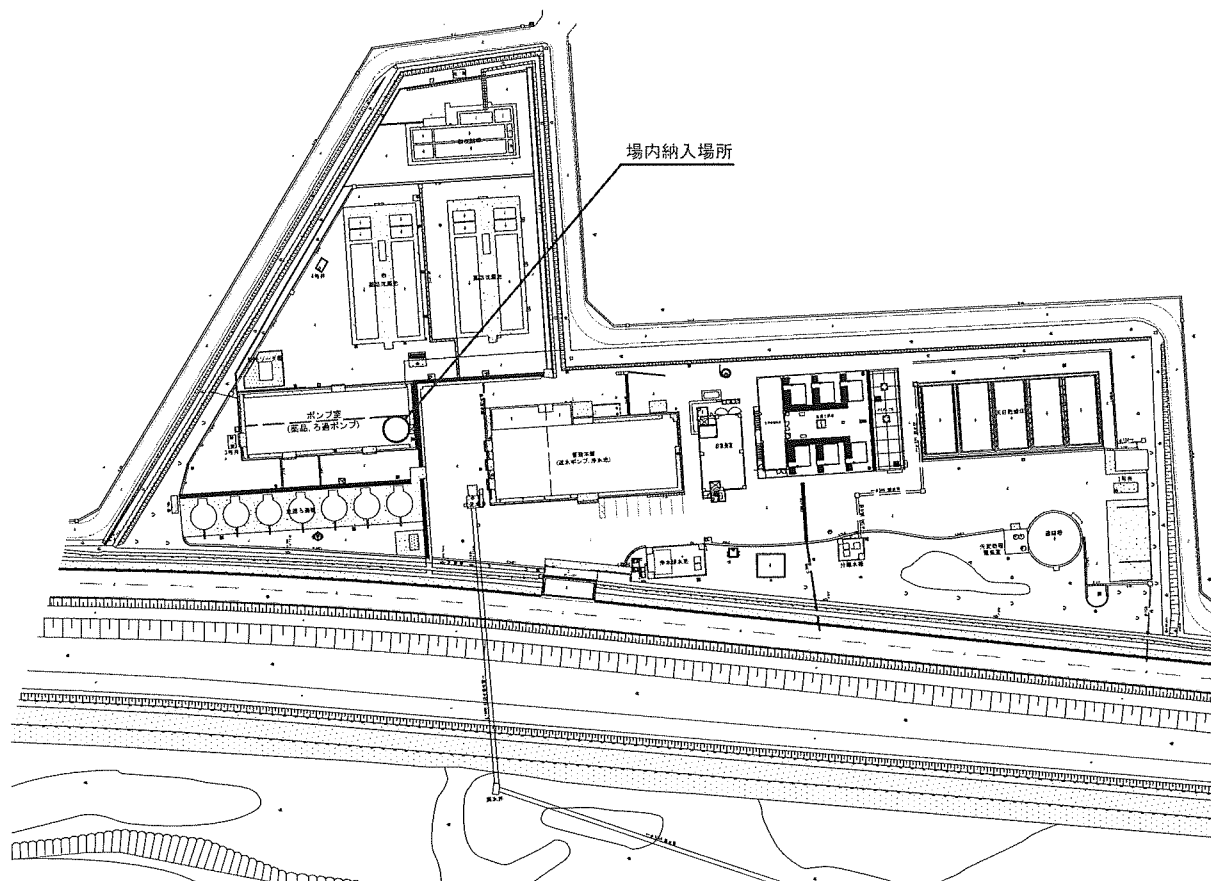
宇治浄水場 場内平面図
