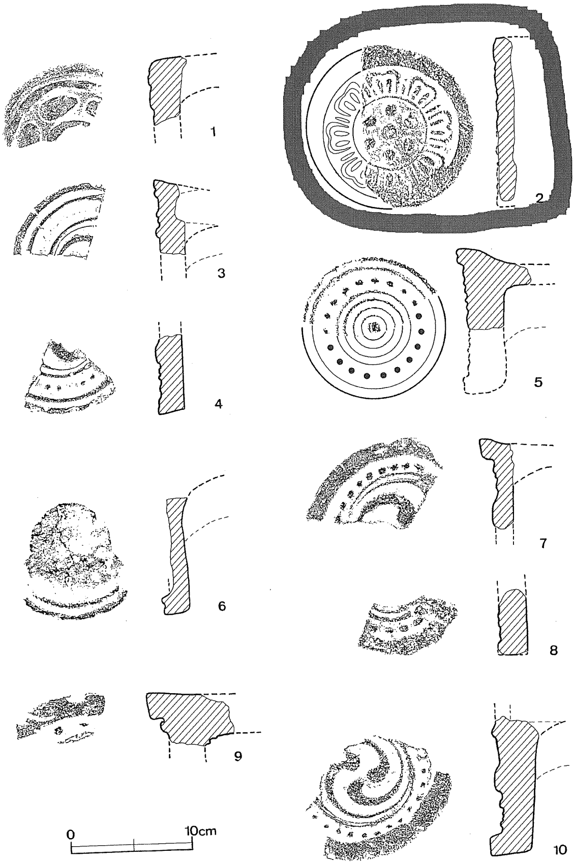
第15図 軒瓦実測図
