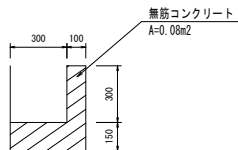
側溝 (3) S=1:25
