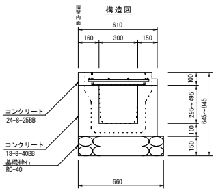
落ちふた式U形側溝3種 取り合い部 (間詰コン有) 参考図 みぞ幅300の場合
