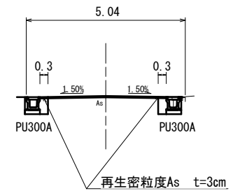
標準断面図 NO. 1
