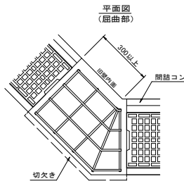
両手掛設置 (参考図)
