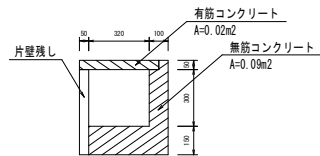
側溝 (1) S=1:25
