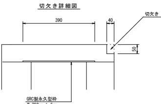
落ちふた式U形側溝3種 取り合い部 (間詰コン有) 参考図 みぞ幅300の場合
