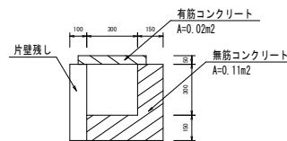
側溝 (2) S=1:25
