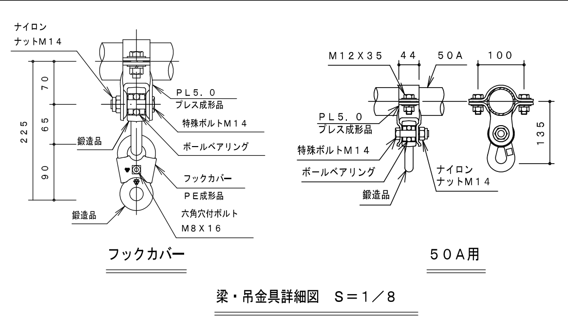
ブランコ修繕詳細図
