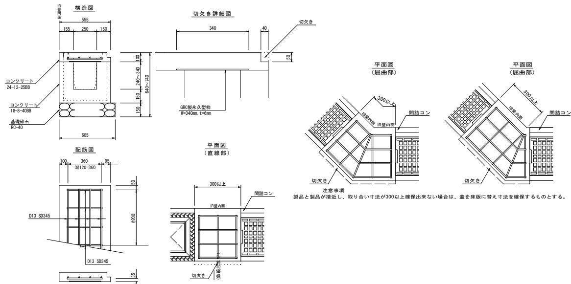
落ちふた式U形側溝3種 取り合い部 (間詰コン有) 参考図 みぞ幅250の場合
