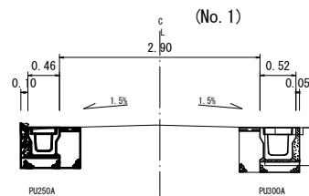
標準横断面 S=1/50
