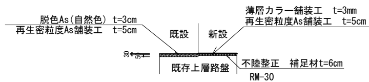
舗装工詳細図 S=1:50
