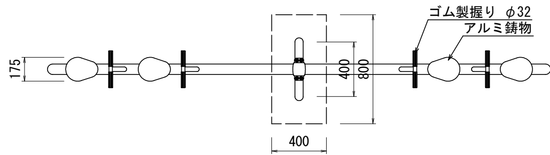
平面図 1:20
