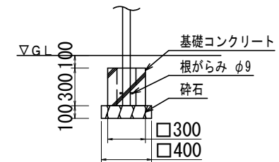
A詳細図 S=1/30
