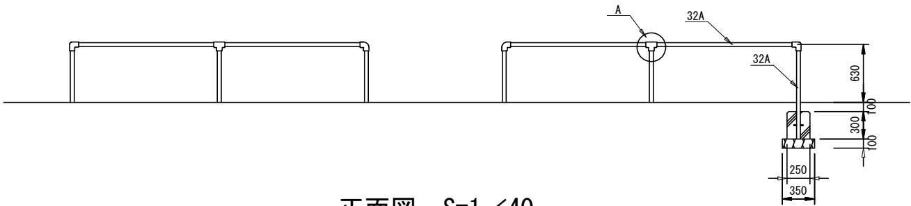
正面図 S=1 / 40
