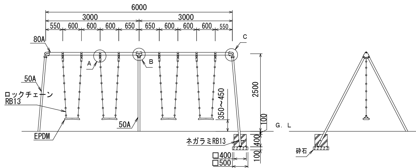
正面図 S=1/50
