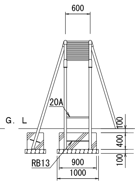
正面図 S=1 / 40
