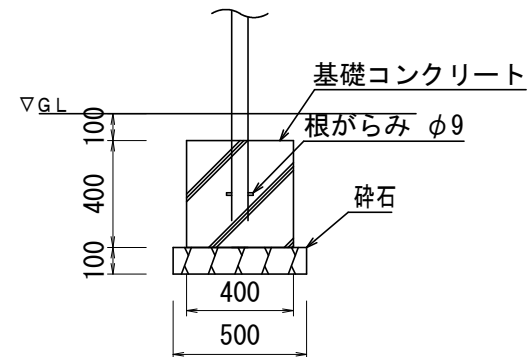
A詳細図 S=1/20
