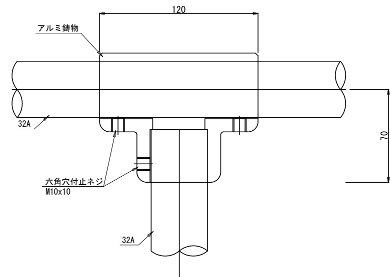
A詳細図 S=1 / 2
