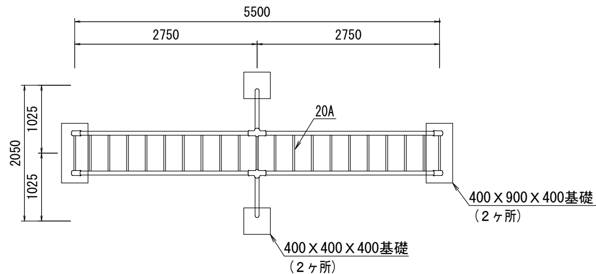
平面図 S=1 : 40
