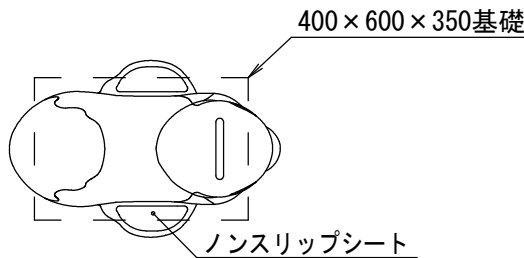
平面図 S=1/15
