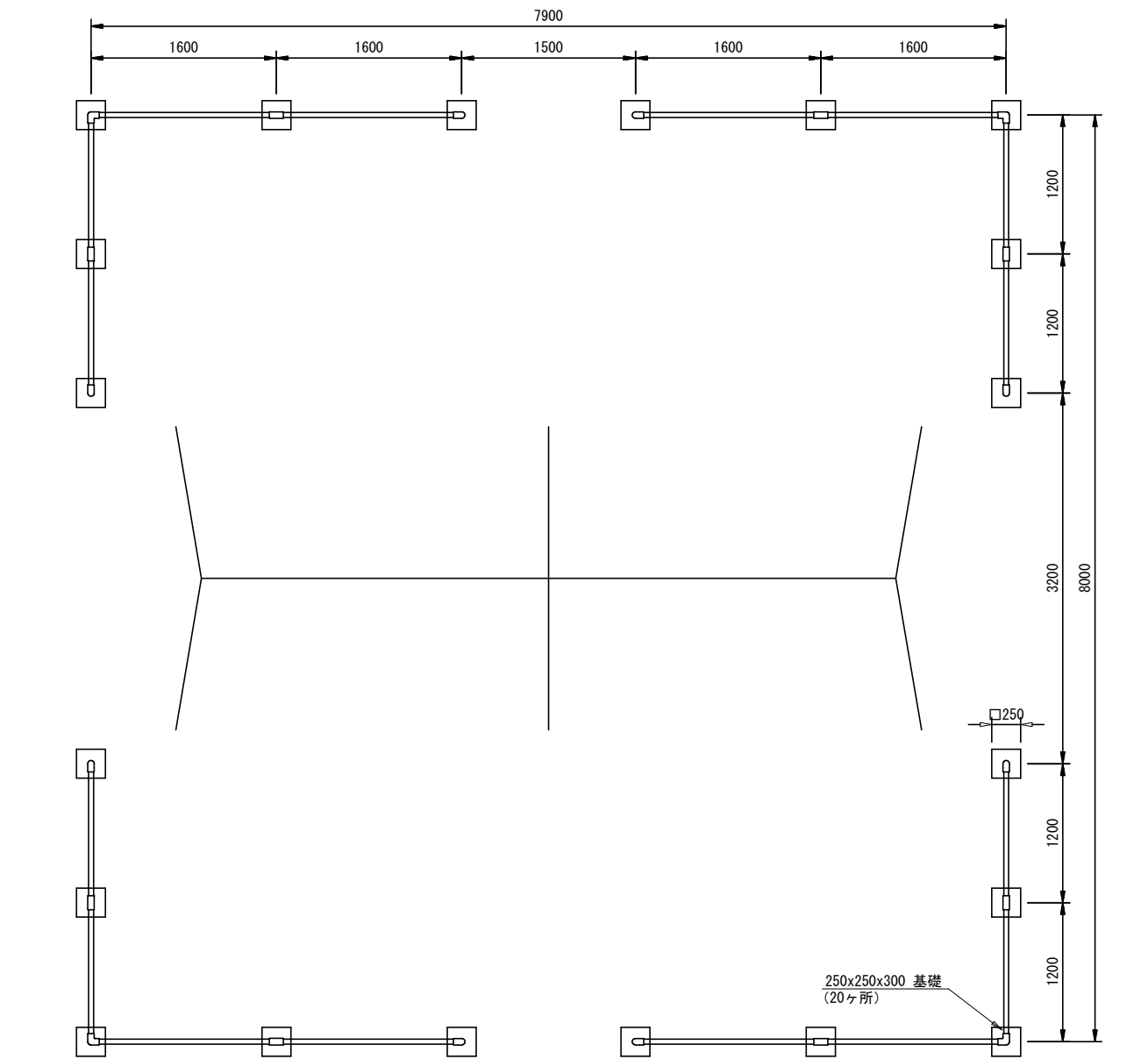
平面図 S=1 : 40
