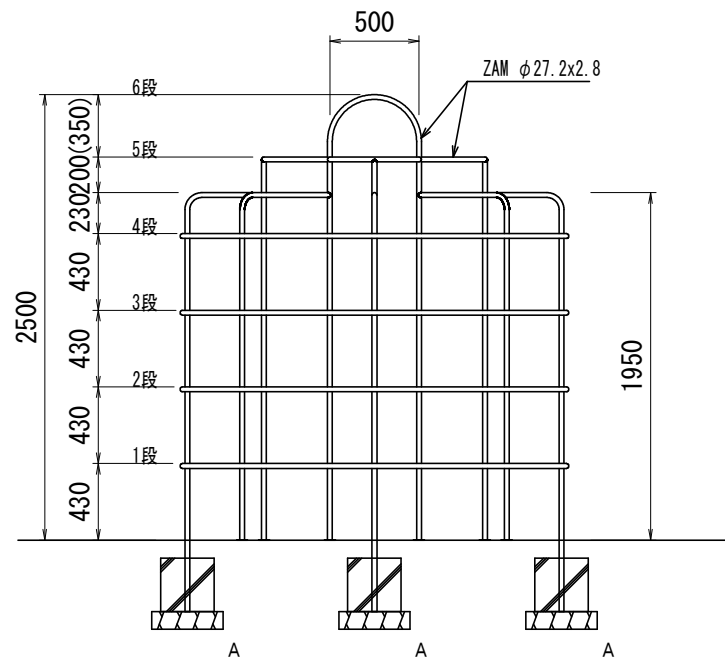
側面図 S=1/30
