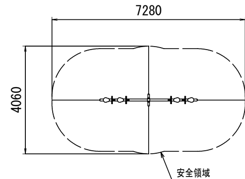
安全領域 1:100
