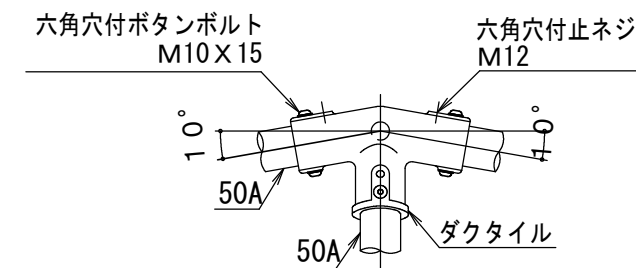
A 詳細図 S=1 / 6
