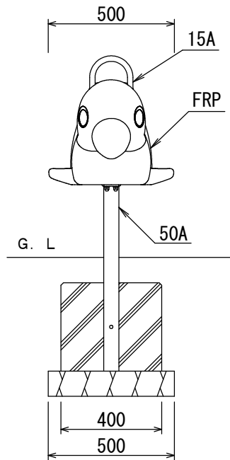
正面図 S=1/15
