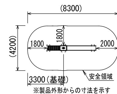
安全領域 S=1/150
