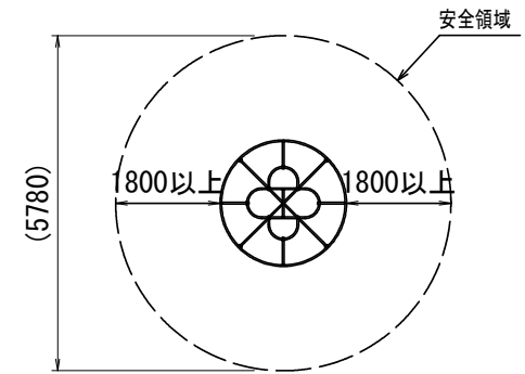
安全領域 S=1/100
