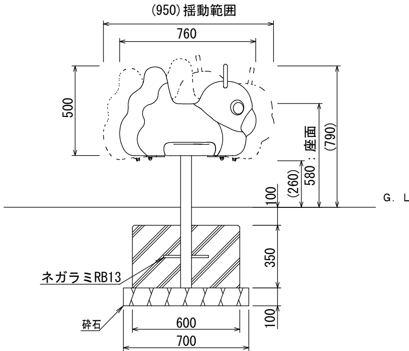
側面図 S=1/15
