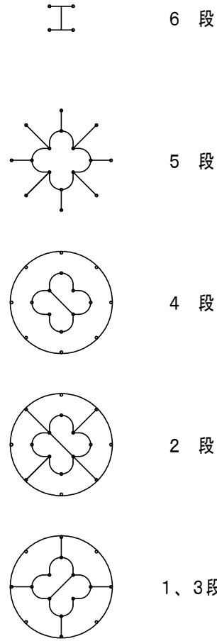
各段平面図
