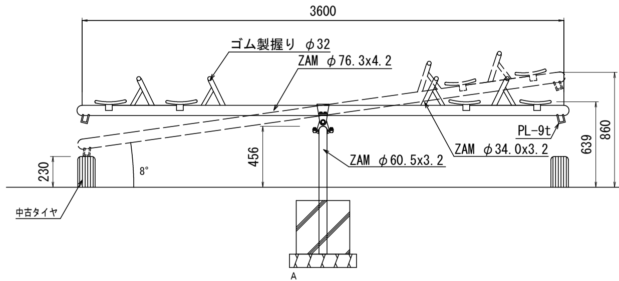
側面図 1:20
