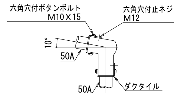
B 詳細図 S=1 / 6
