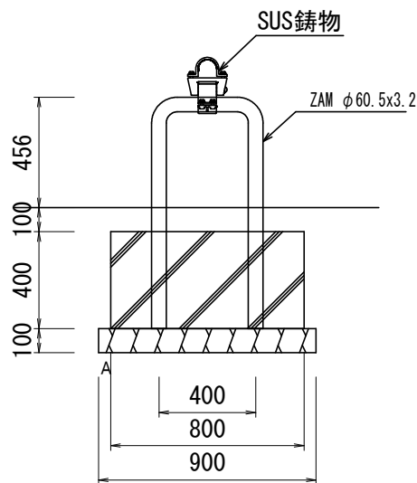
正面図 1:20
