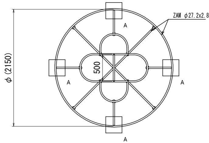
平面図 S=1/30
