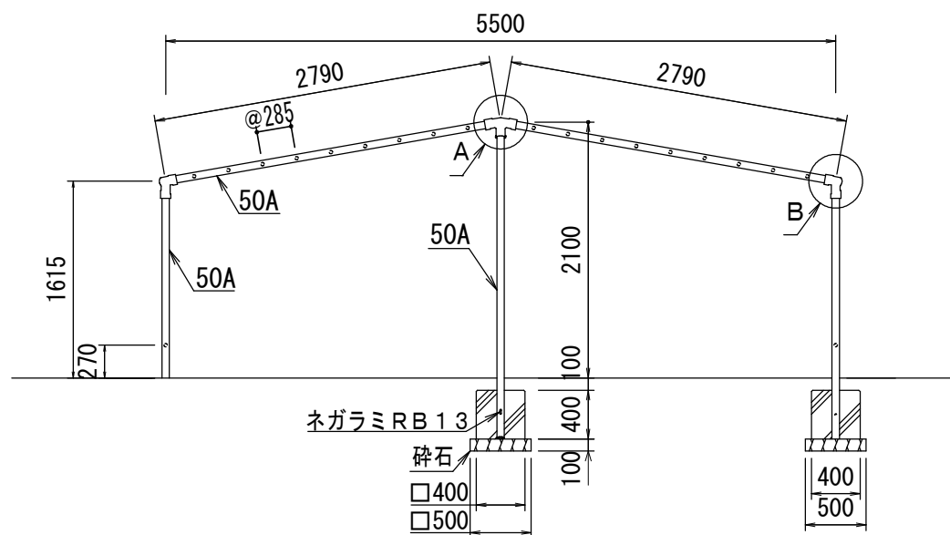
側面図 S=1 / 40
