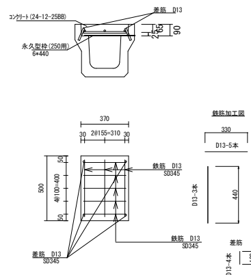
ずれ止め床版工250
