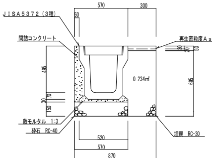
側溝 P U 3 0 0 B
