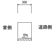
標準ベース修正工
