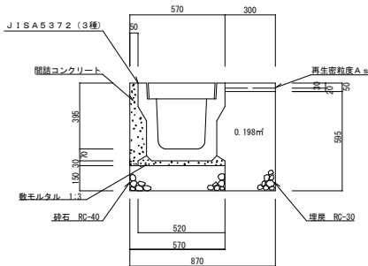
側溝 P U 3 0 0 A
