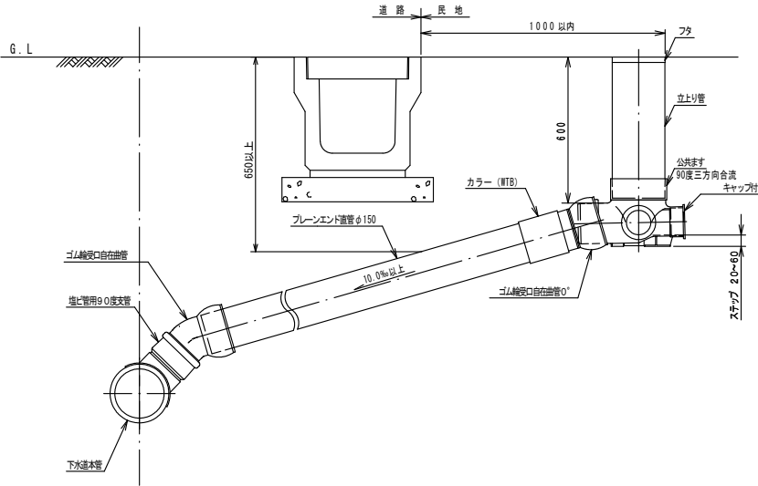
ます径200 横型 公共汚水ます標準図
