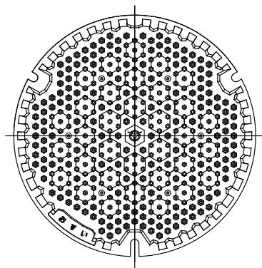
断面図
