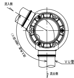
平面图
