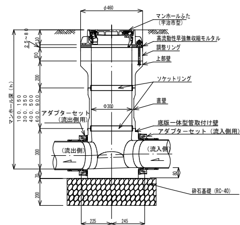
A-A 断面図
