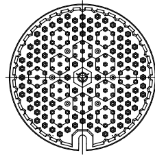
ふた平面図
