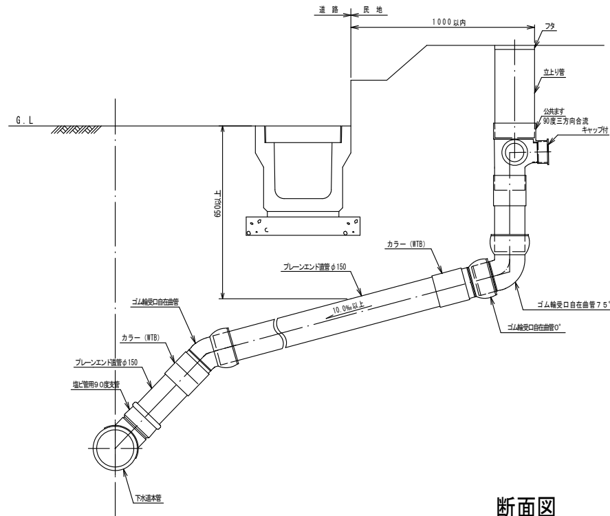
ます径200 縦型 公共汚水ます標準図
