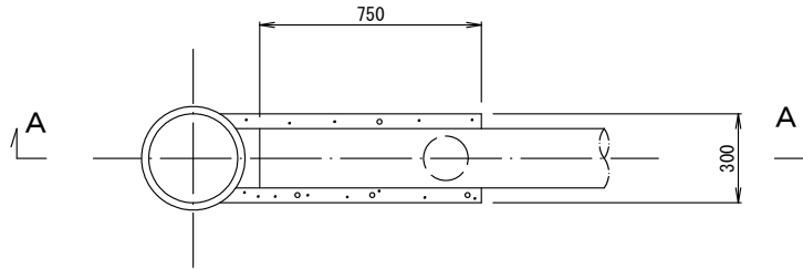
平面図
