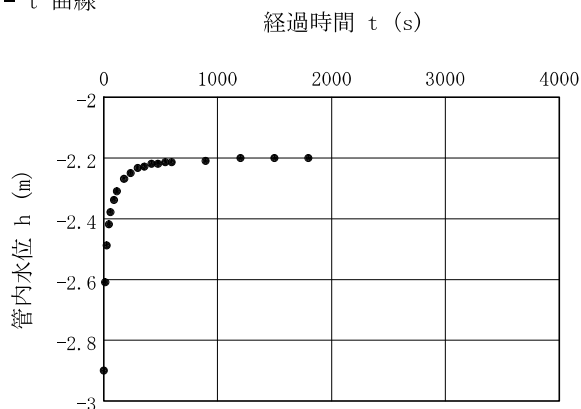
h - t 曲線
