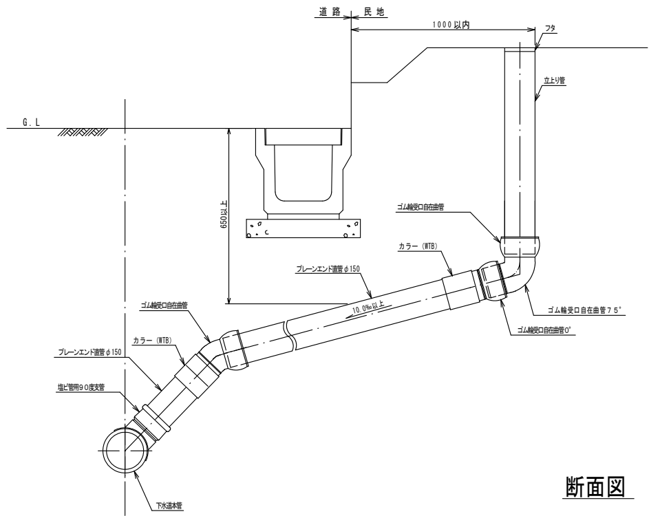
ます径150 縦型 特殊公共汚水ます縦型標準図
