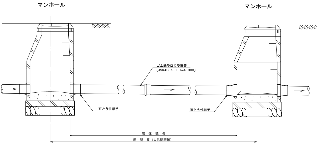
縦断図
