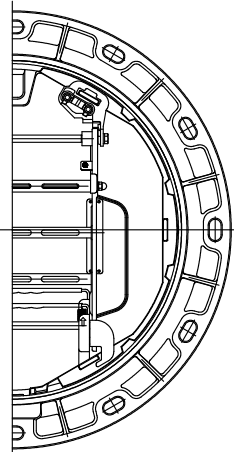
受枠平面図
