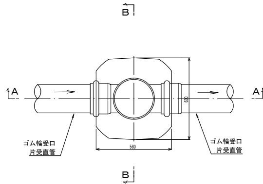
平面图
