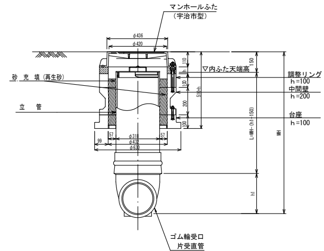
B-B断面図
