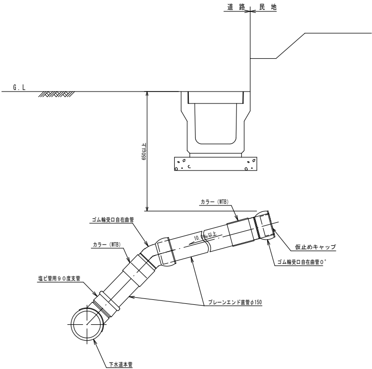
取付管止め標準図
