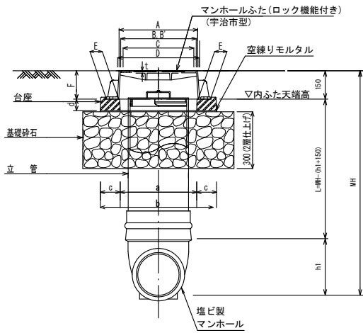
B-B断面図
