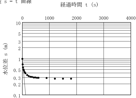
log s - t 曲線
