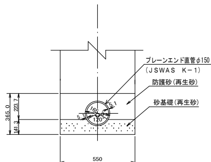
断面図
