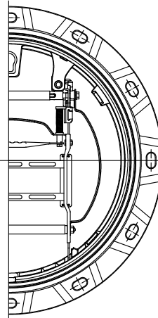
受枠平面図
