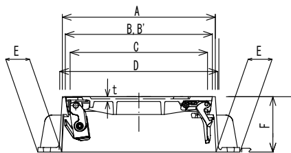
【標準型防護ふたT-25, T-14 寸法表】
