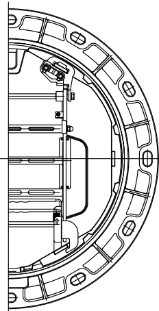
受枠平面図
