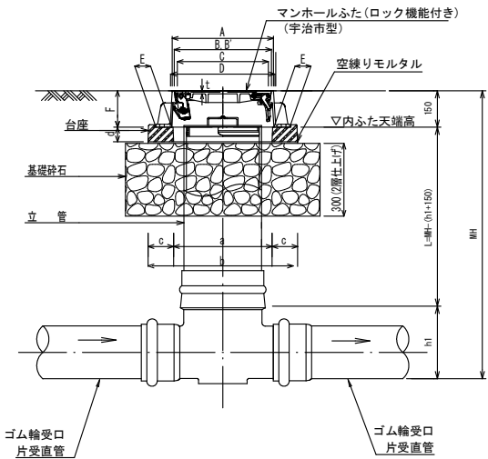
A-A断面図
