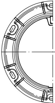
受枠平面図
