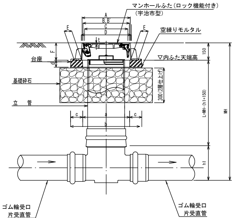
A-A断面図
