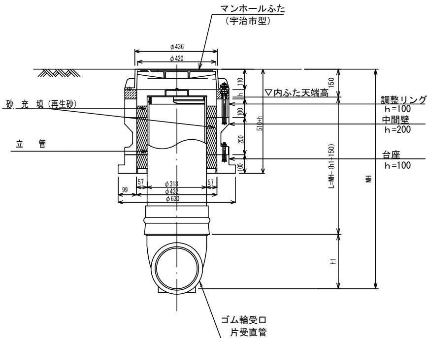
B-B断面図
