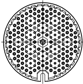
ふた平面図
