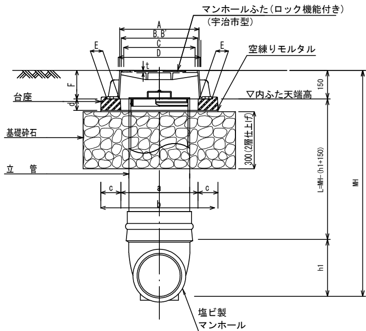
B-B断面図
