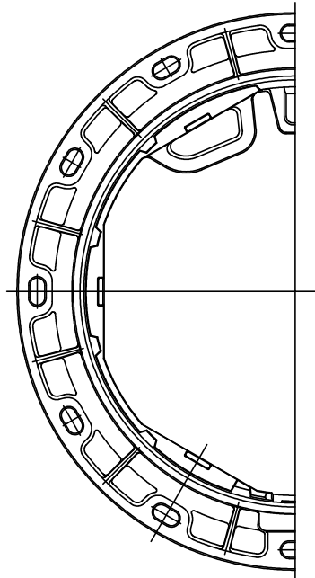
受枠平面図
