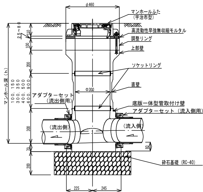
A-A断面図
