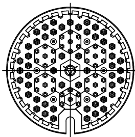
ふた平面図
