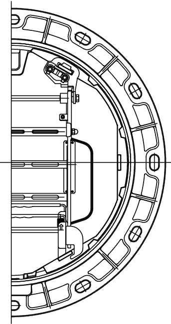
受枠平面図
