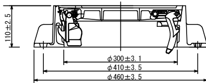
断面図
