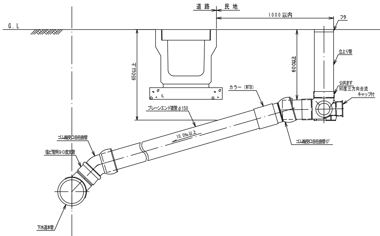
断面図
