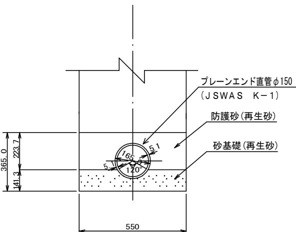
断面図
