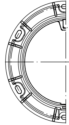
受枠平面図
