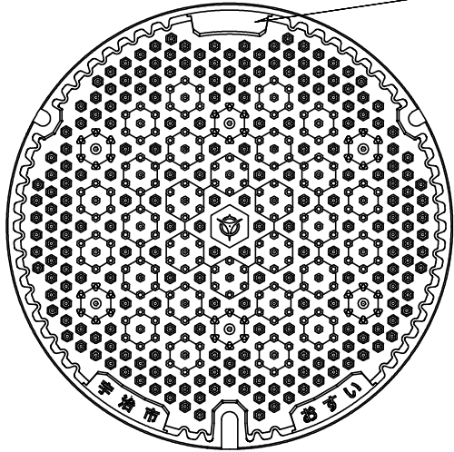
ふた平面図
