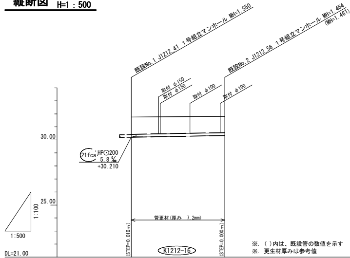
縦断面図 V=1 : 100 H=1 : 500
