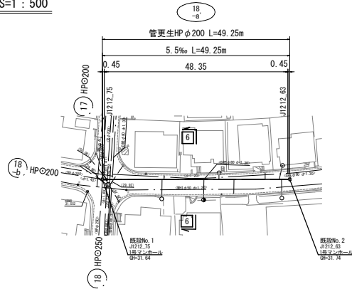
縦断面図 V=1:100 H=1:500
