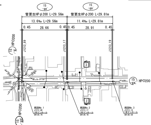
平面図 S=1 : 500
