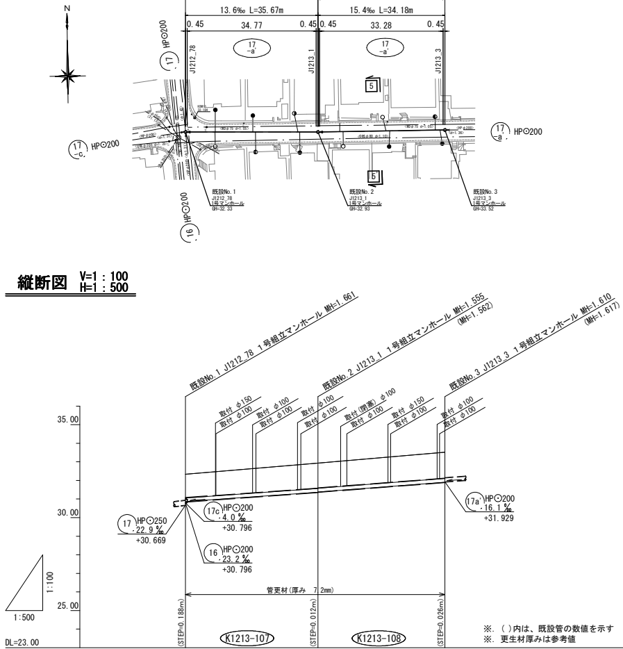
平面图 S=1 : 500
