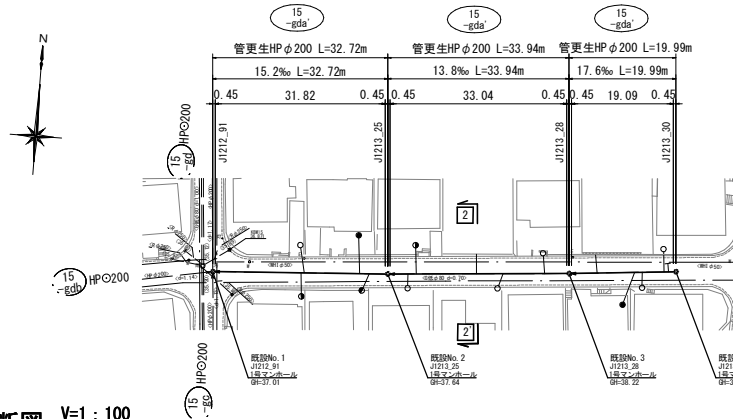
縦断面図 V=1:100 H=1:500
