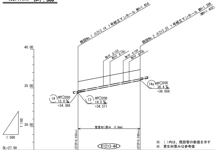
縦断面図 V=1:100 H=1:500
