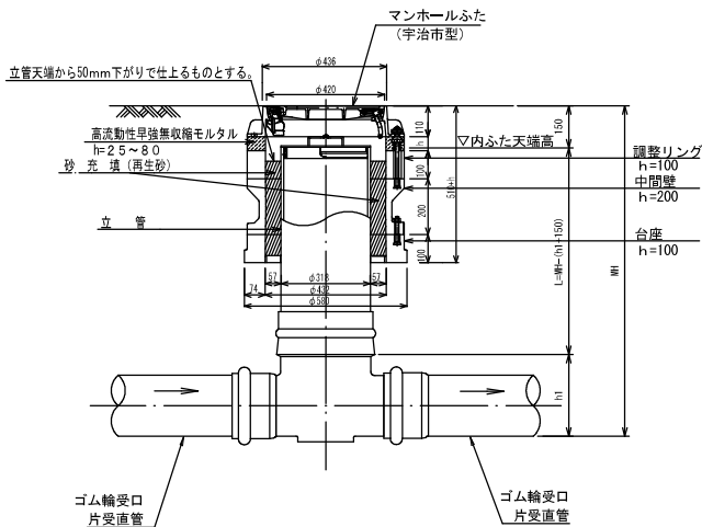
A-A断面図
