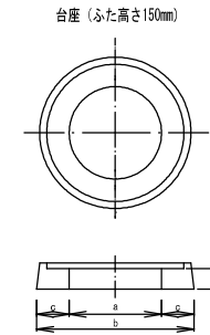
【標準型台座PB25A、RB25A（ふた高さ150mm）寸法表】
