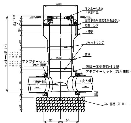
A-A断面図
