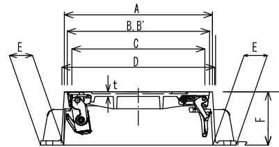
【標準型防護ふたT-25、T-14 寸法表】
