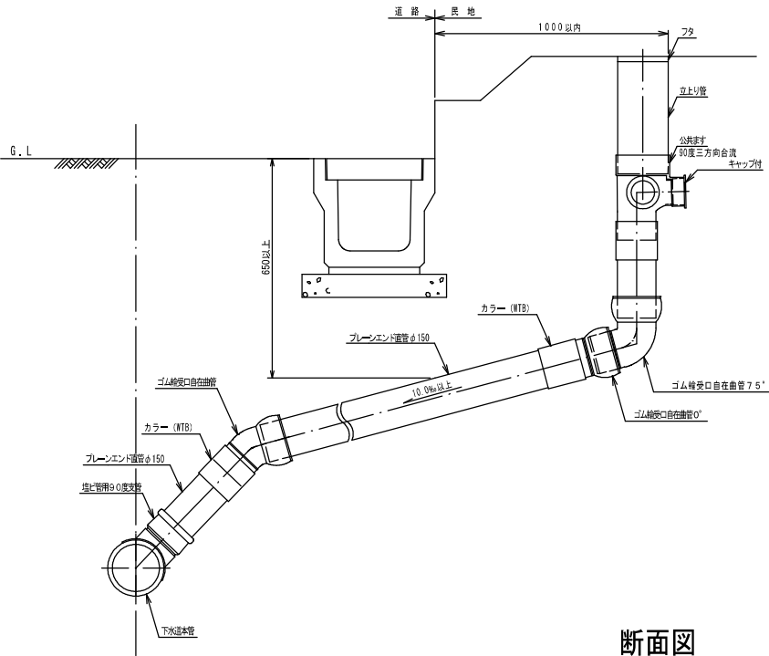
ます径200 縦型 公共汚水ます標準図
