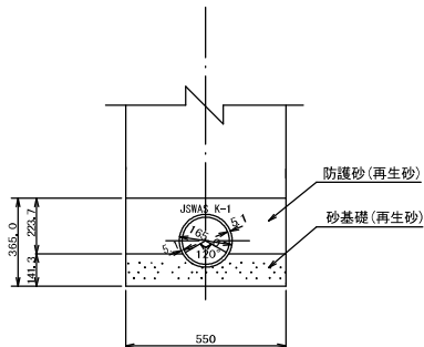
断面図
