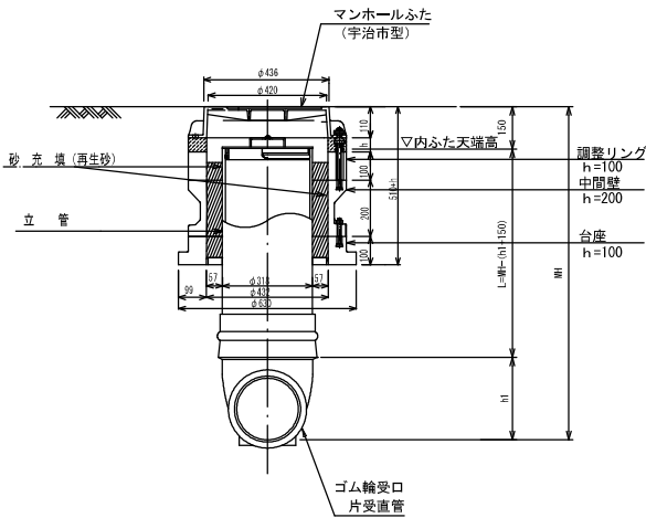
B-B断面図
