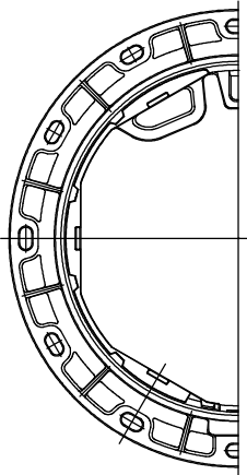
受枠平面図
