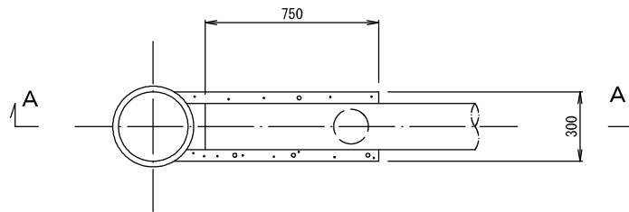
平面图
