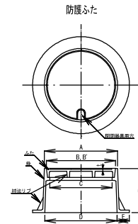
【標準型防護ふたT-25、T-14 寸法表】
