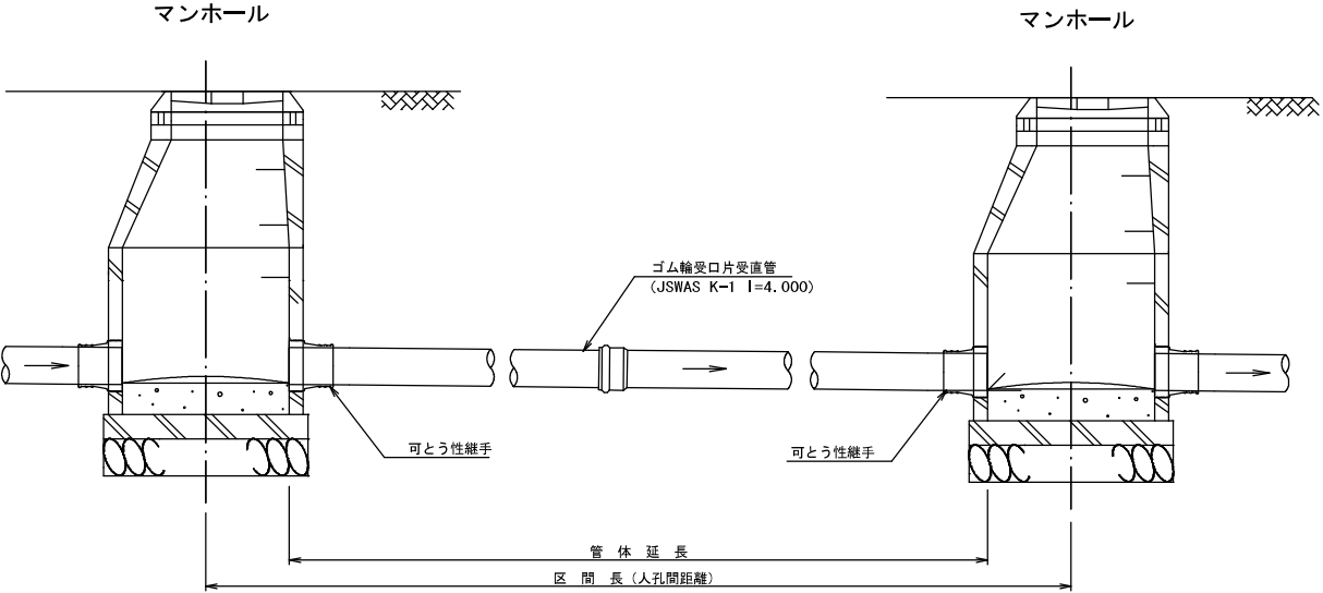
縦断図
