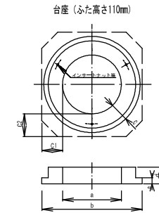
【標準型台座RBA, CBA (ふた高さ110mm) 寸法表】
