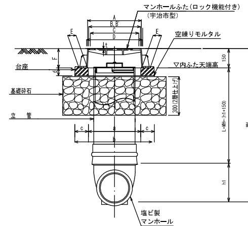
B-B断面图
