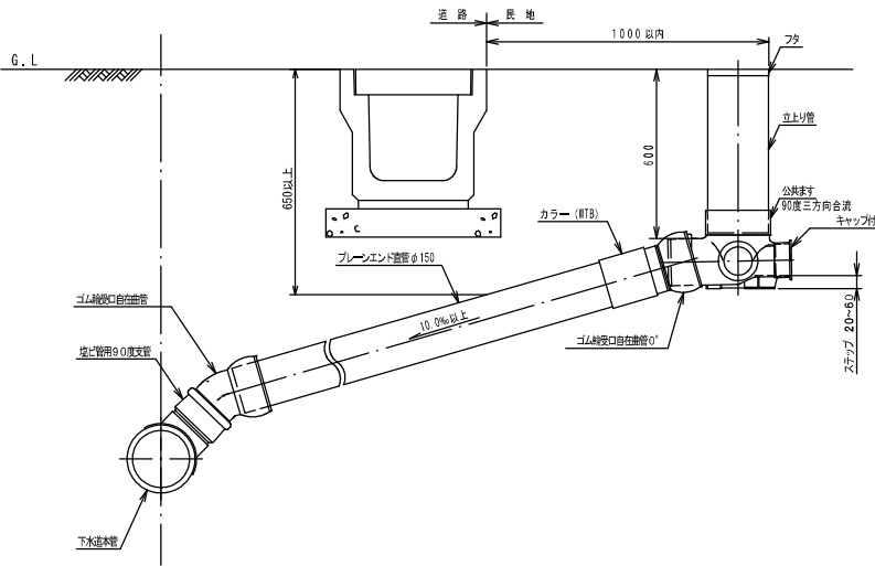
ます径200 横型 公共汚水ます標準図
