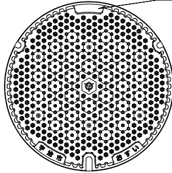
ふた平面図
