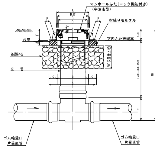
A-A 断面図
