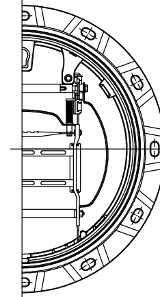
受枠平面図
