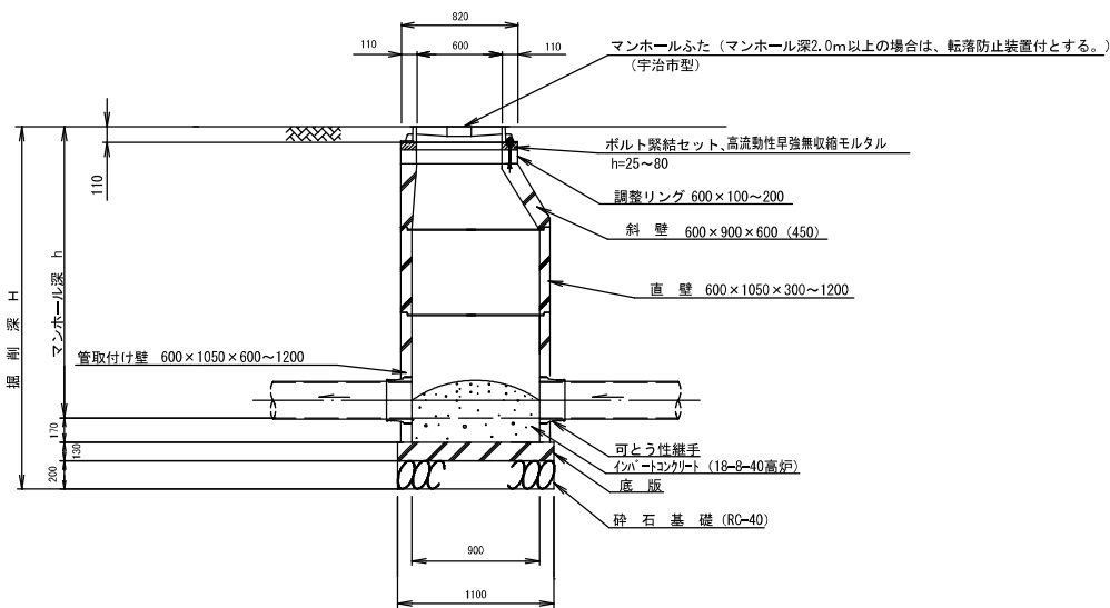
A-A断面図
