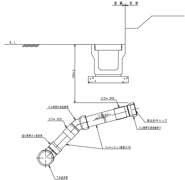
取付管止め標準図
