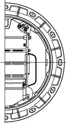
受枠平面図
