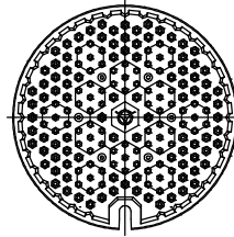
ふた平面図
