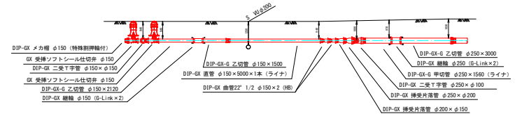
G - G 断面
