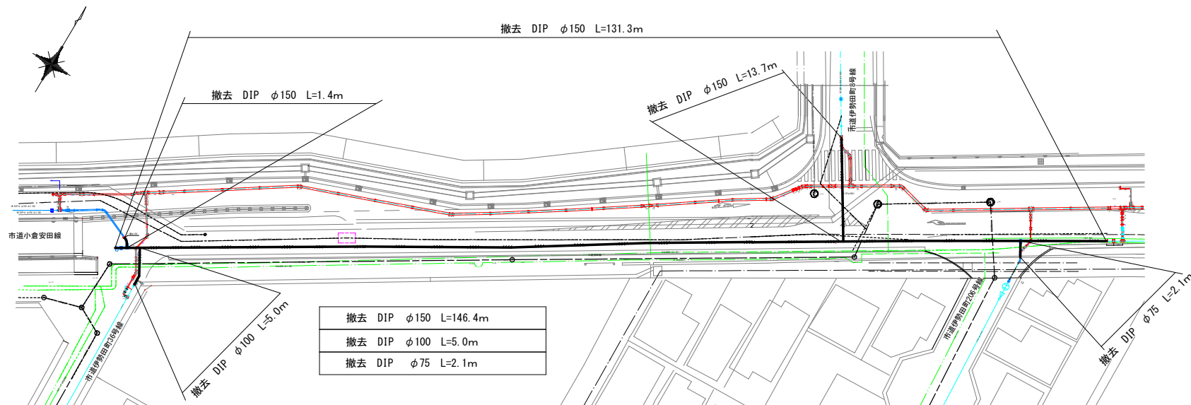
撤去図 S=1/250
