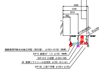
H - H 断面
