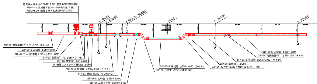
E - E 断面
