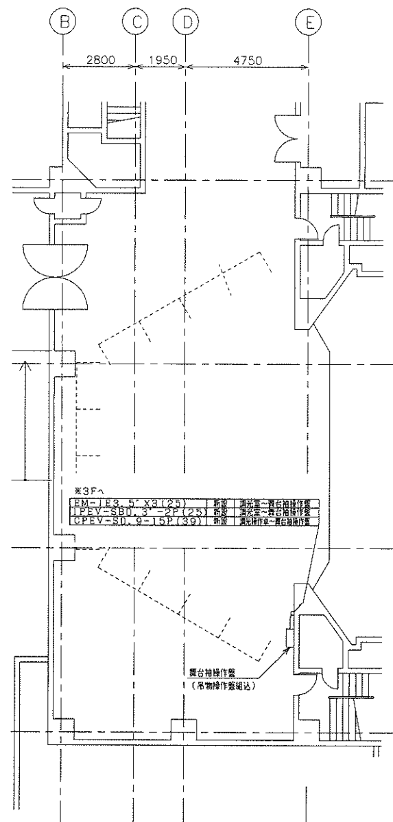
1F平面図
