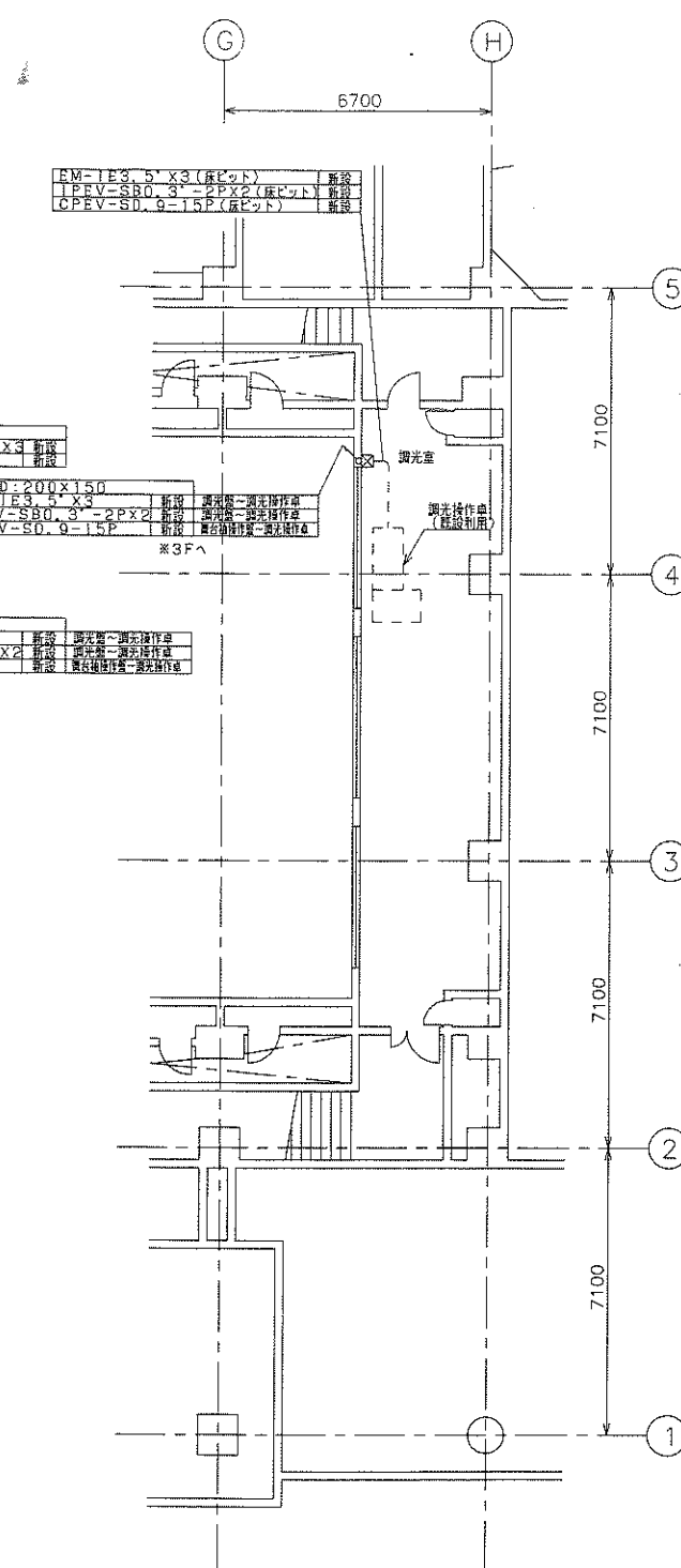
M3F平面図
